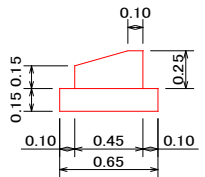
基礎構造図 1/50
