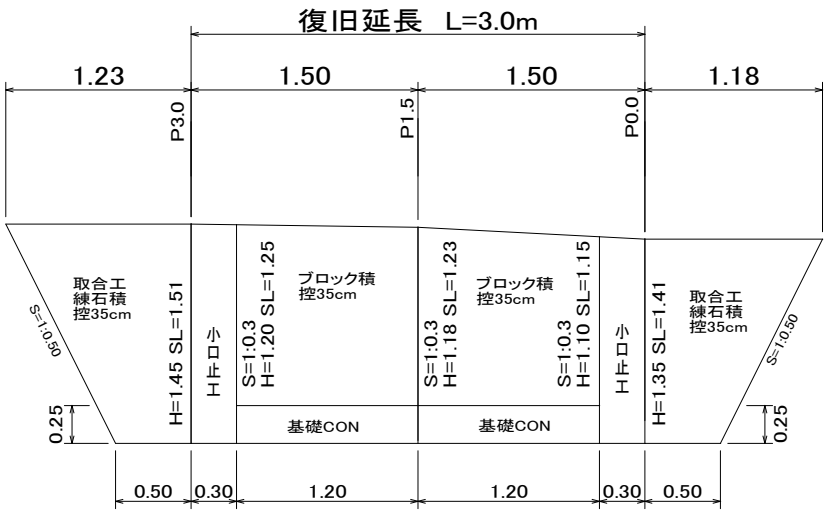
擁壁展開図 1/50
