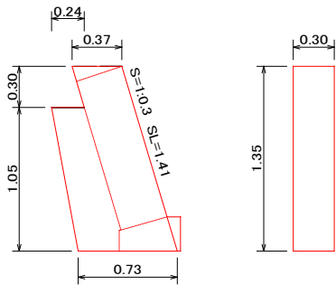
小口止 1/50
