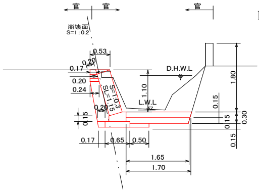
横断面図 1/100
