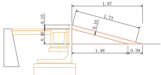
乗入工正面図
