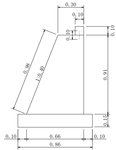
小型擁壁構造図
