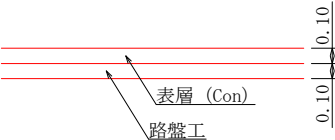
既設Con舗装構成図 1/50
