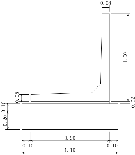
L型擁壁構造図
