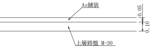
舗装構成図
