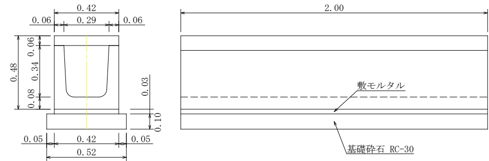
横断側溝構造図 (300×400)
