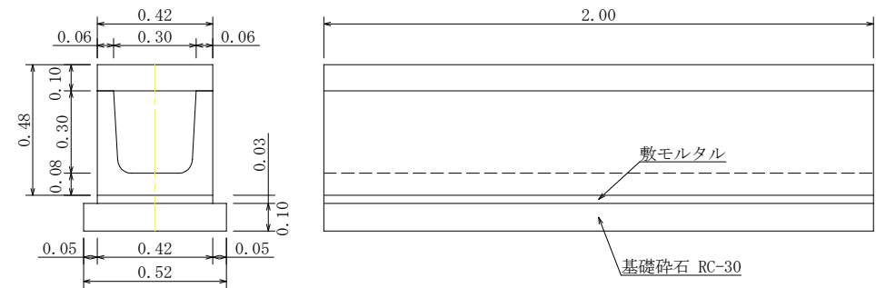
縦断側溝構造図 (300×300)
