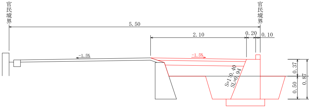
⑤—⑤断面
