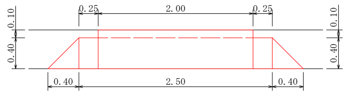
乗入工正面図
