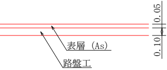
既設As舗装構成図 1/50
