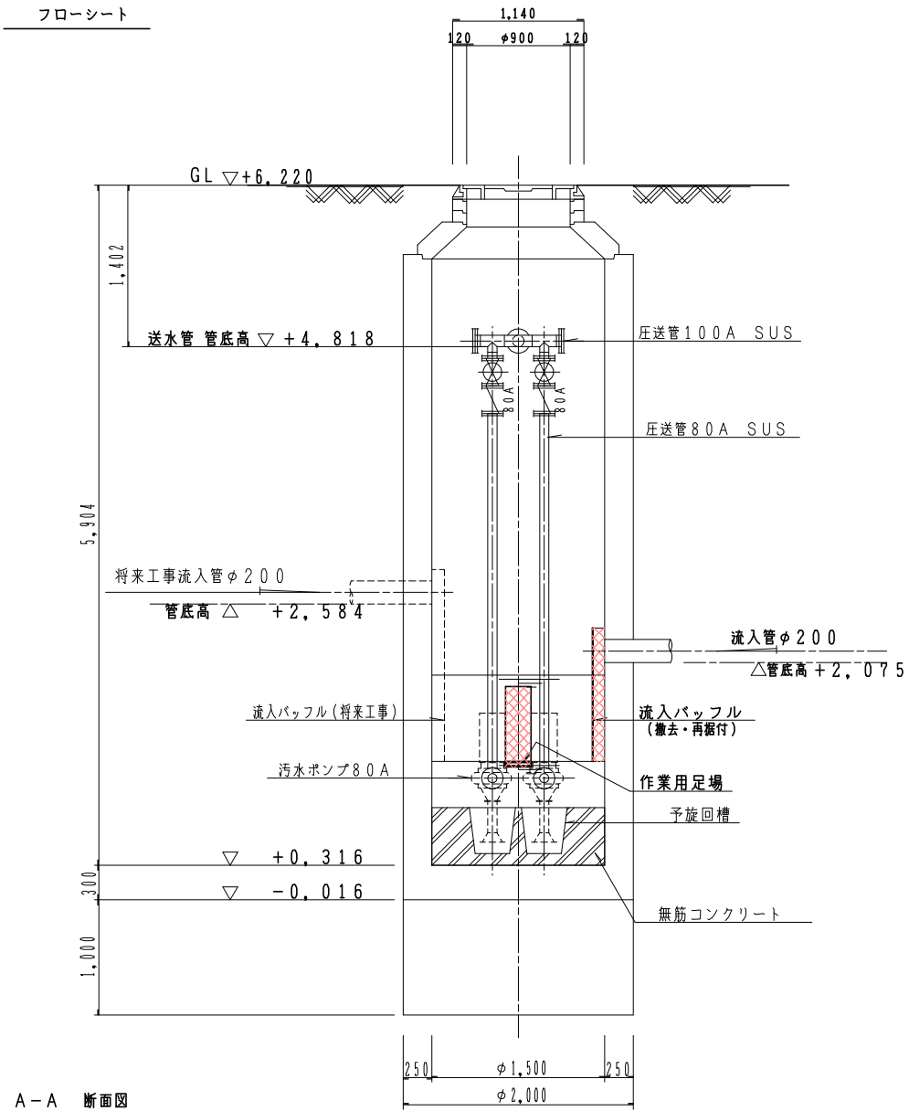
フローシート
