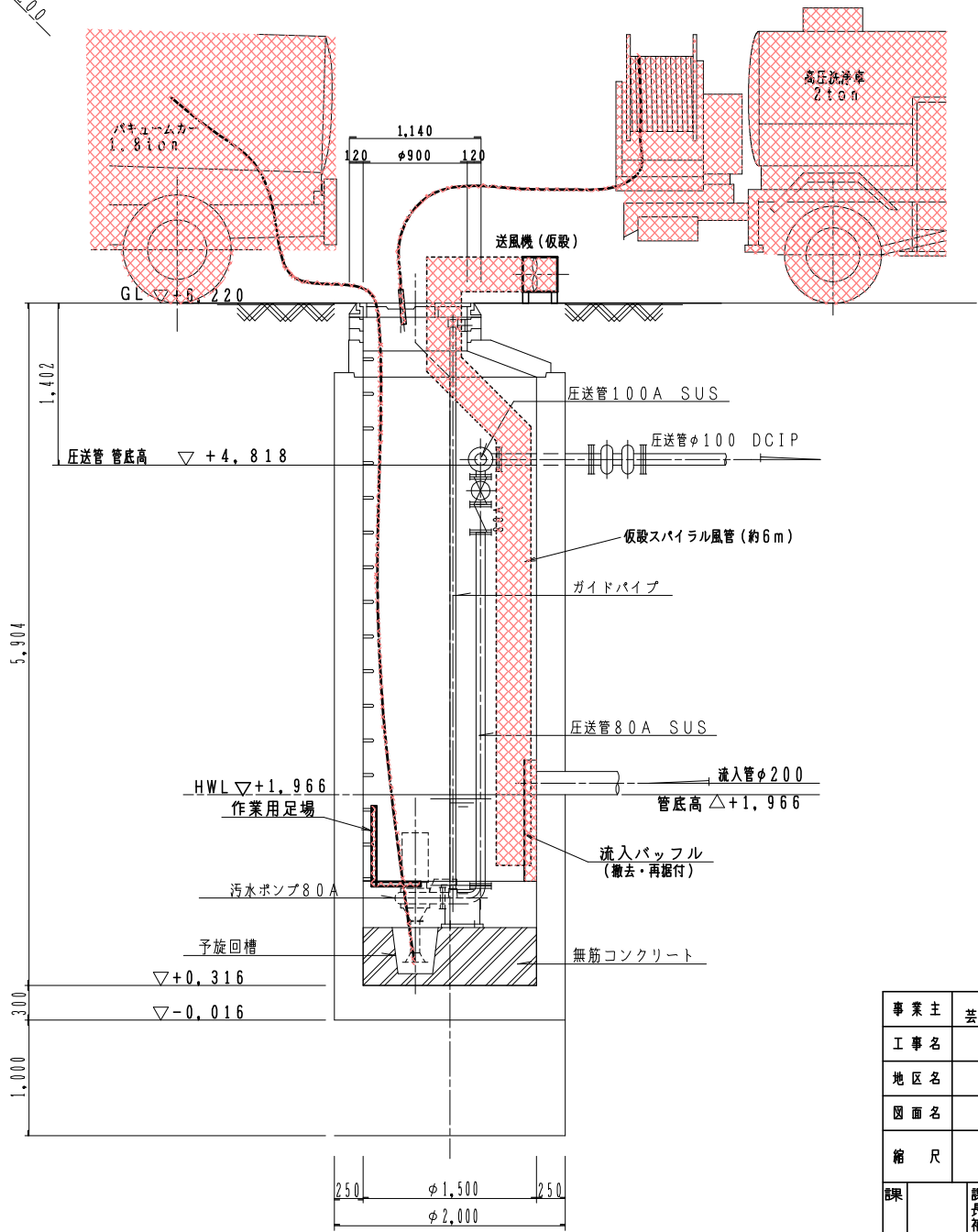
B-B 断面図
