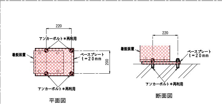
アンカーボルト詳細図 1/10
