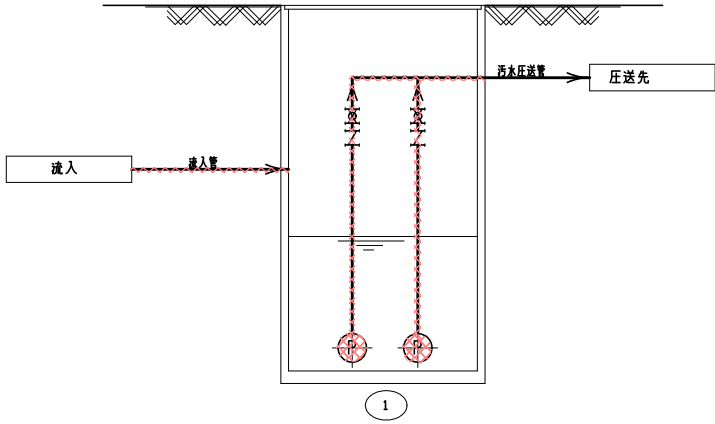
フローシート
