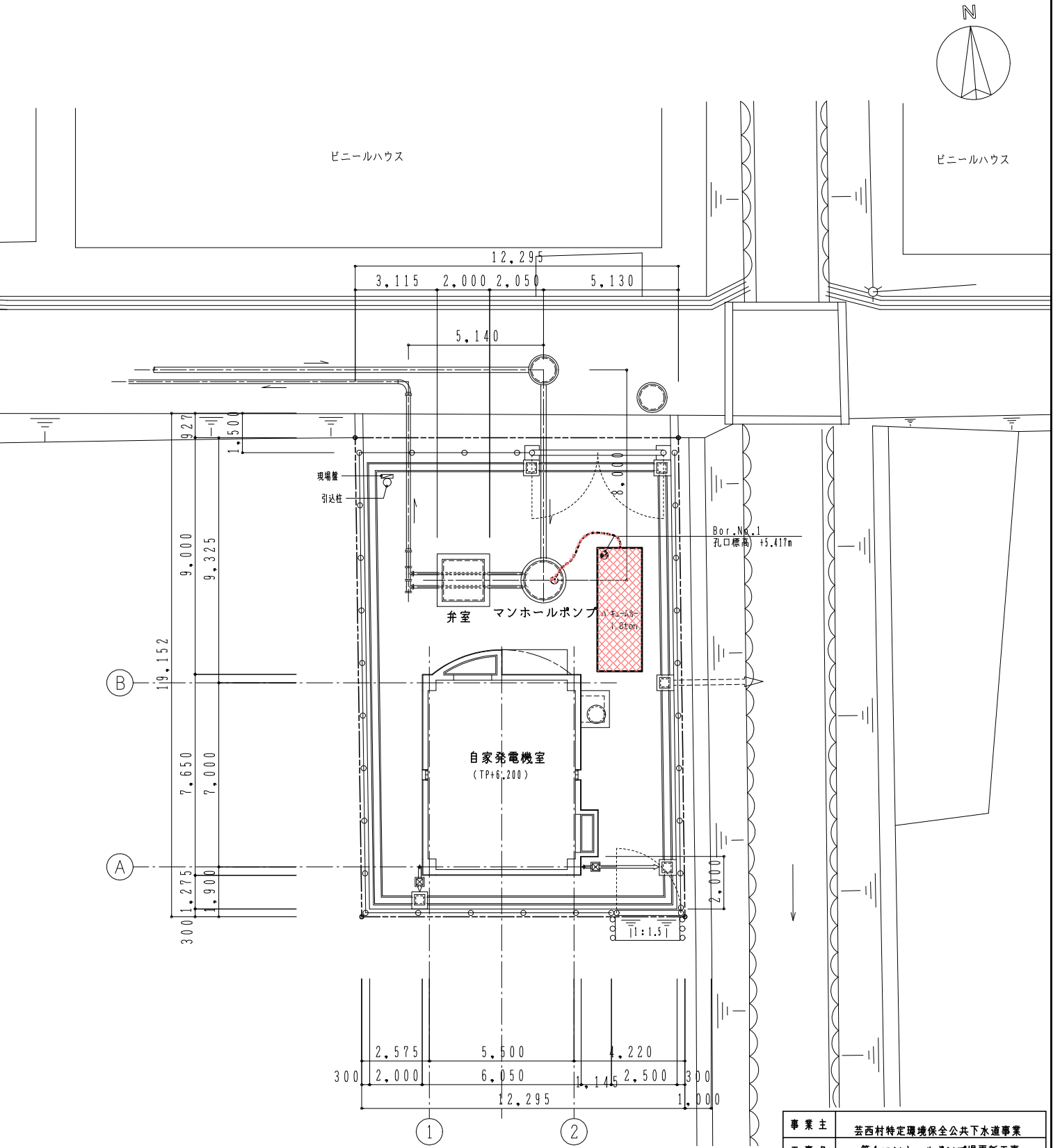
西分中継ポンプ場 一般平面図 S=1/100
