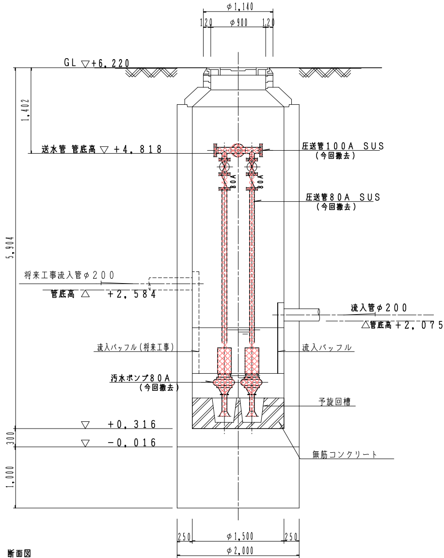
A-A 断面図
