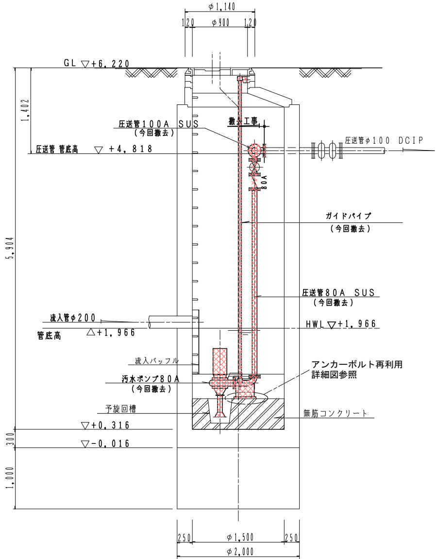
B-B 断面図
