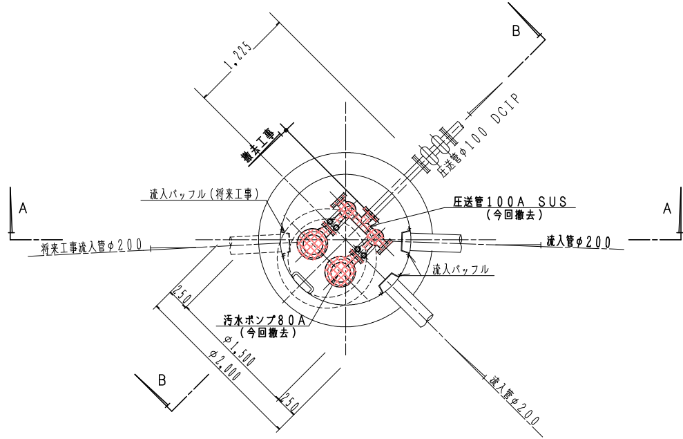
平面図
